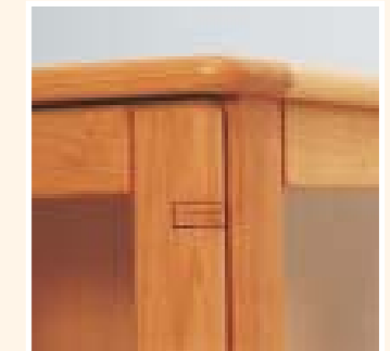
Handwerklich ausgereifte Holztürbänder für einen Öffnungswinkel von über 180 Grad
